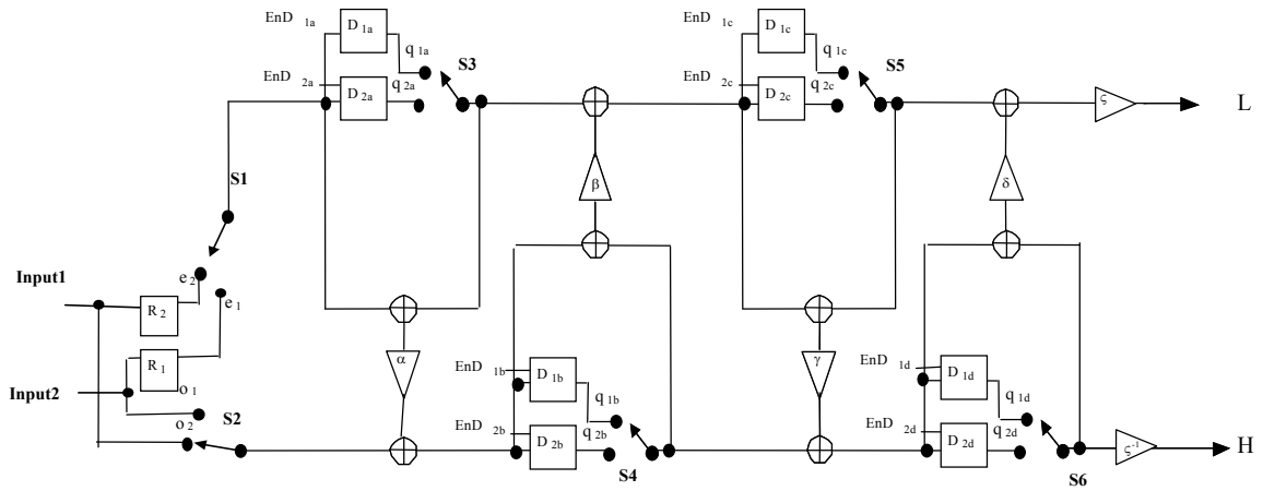
Figure 28. The DSA PE Circuit for the 9/7 DWT.
