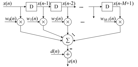
Fig. 3. Error computation module.
