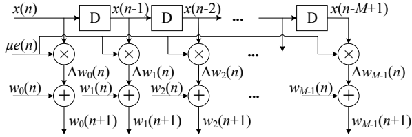
Fig. 4. Weight update module.
